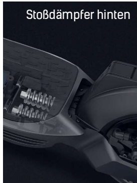
Scheibenbremse hinten und Kennzeichenhalter
